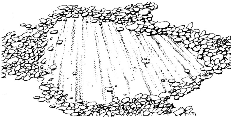
Gletscherkritzungen
