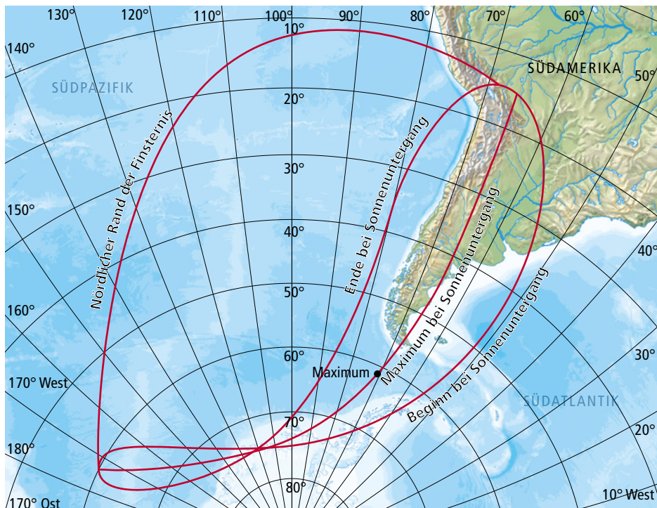
F.1 Sichtbarkeitsgebiet der partiellen Sonnenfinsternis vom 30. April 2022
