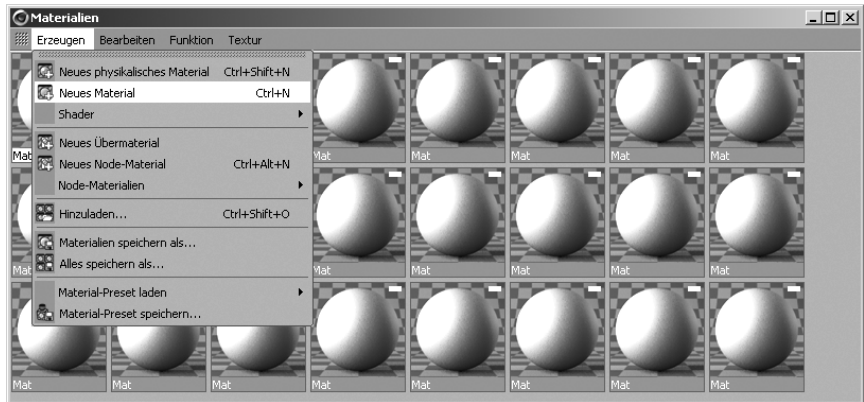
Abbildung 1.7 Der Material-Manager
