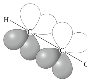
zwei \pi -Bindungen (senkrecht zueinander)
