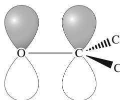
Seitenansicht der \pi -Bindung
