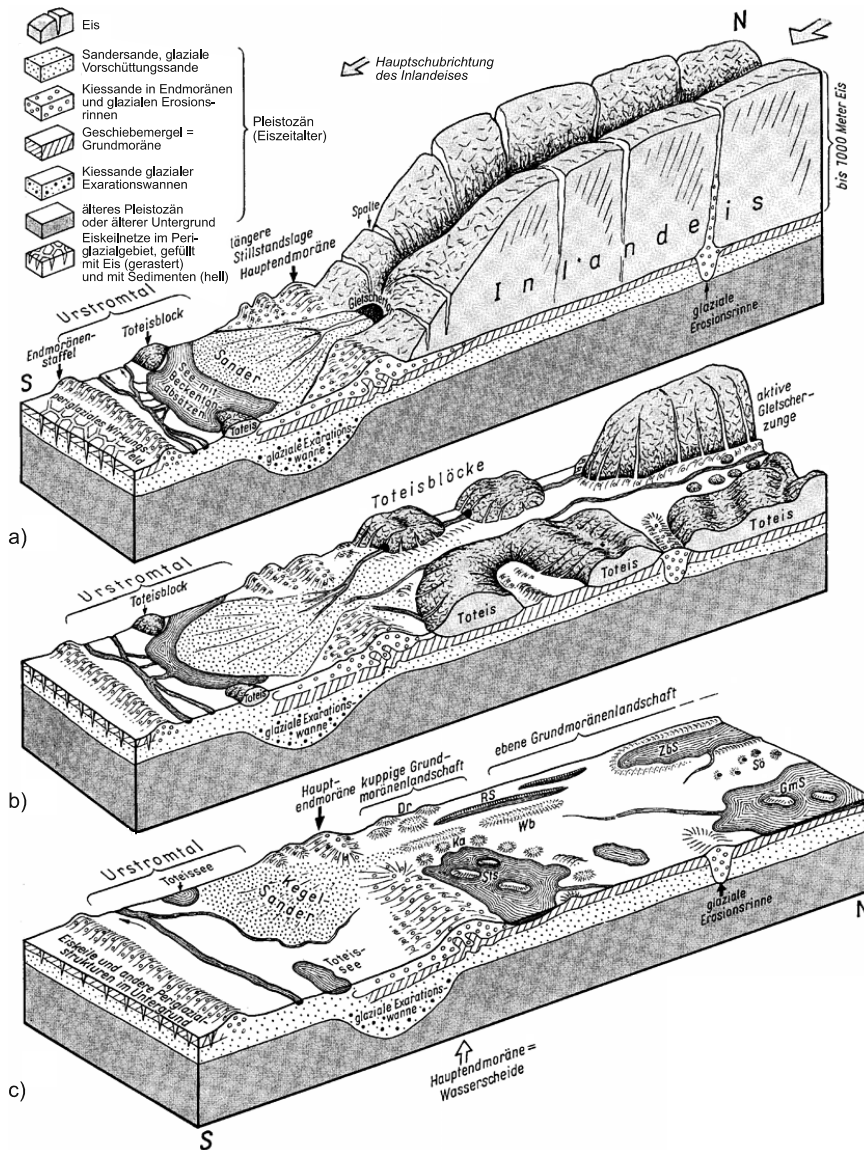
Bild 1-4 Formung der Landschaft des Norddeutschen Tieflands durch das eiszeitliche Inlandeis (aus [251])
