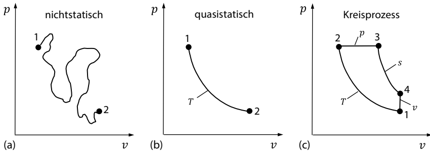
Abb. 2.6 Zustandsänderungen im p, v -Diagramm.
