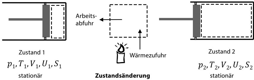
Abb. 2.5 Zustandsänderung eines geschlossenen Systems.
