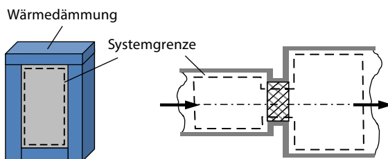
Abb. 2.2 Adiabate Systeme.
