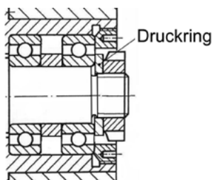
Bild 1.15 Axiales Verspannen der Kugellagerinnenringe
