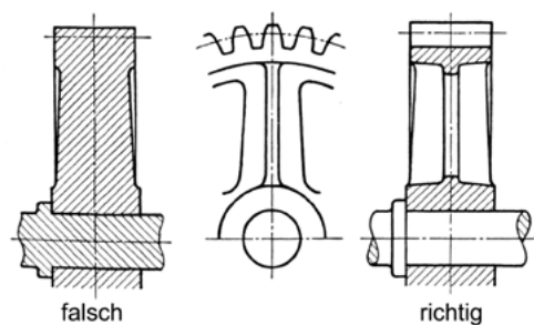
Bild 1.2 Falsche und richtige Schnittdarstellung an Zahnrad und Welle [43]
