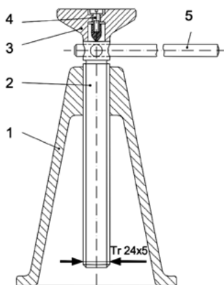
Bild 1.11 Schraubenwinde
