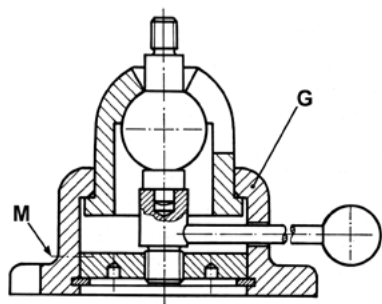
Bild 1.13 Kugelpopf [34]
