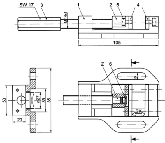
Bild 1.14 Maschinenschraubstock
