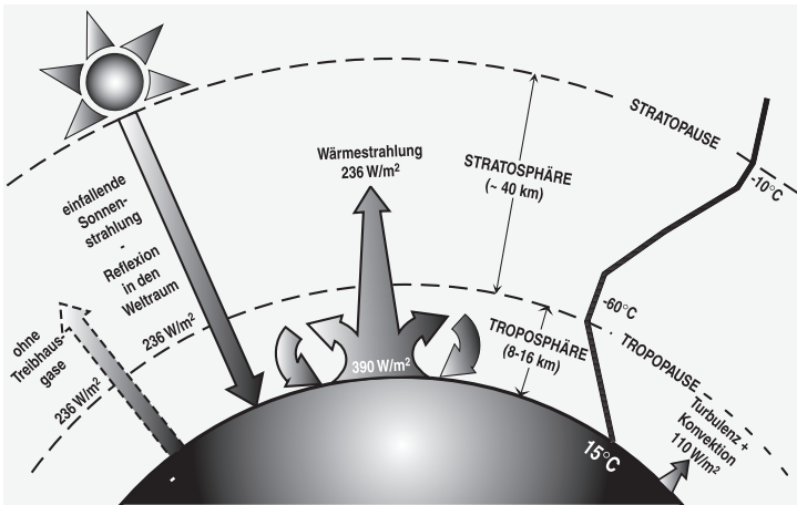
Abb. 2: Der natürliche Treibhauseffekt der Erde
