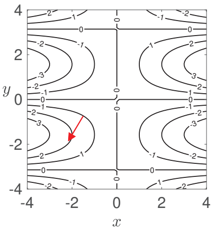
Bild 1.14 Höhenlinien zu f(x, y) = x \sin y mit eingezeichnetem Gradienten an der Stelle (-1.5, \arcsin(-\frac{2}{3}))
