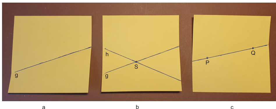
Bild 1.1 Faltgeraden
