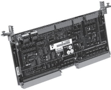
Bild 1.5 Digitale Regelungsbaugruppe für einen Gleichstromantrieb
