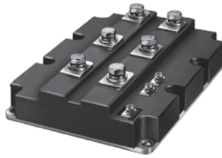
Bild 1.6 Hochleistungs-IGBT (Insulated Gate Bipolar Transistor) für Frequenzumrichter
