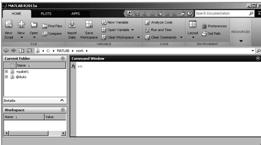
Bild 1.3 MATLAB-Desktop
