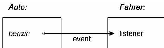
Bild 1.2 Ereignis ( event ) als Nachricht an den „ listener “
