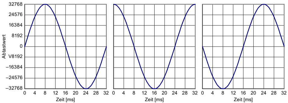
BILD 2.3 Sinusschwingungen mit den Phasenlagen 0, 90, 180° (im Bogenmaß: 0, \frac{\pi}{2} , \pi )
