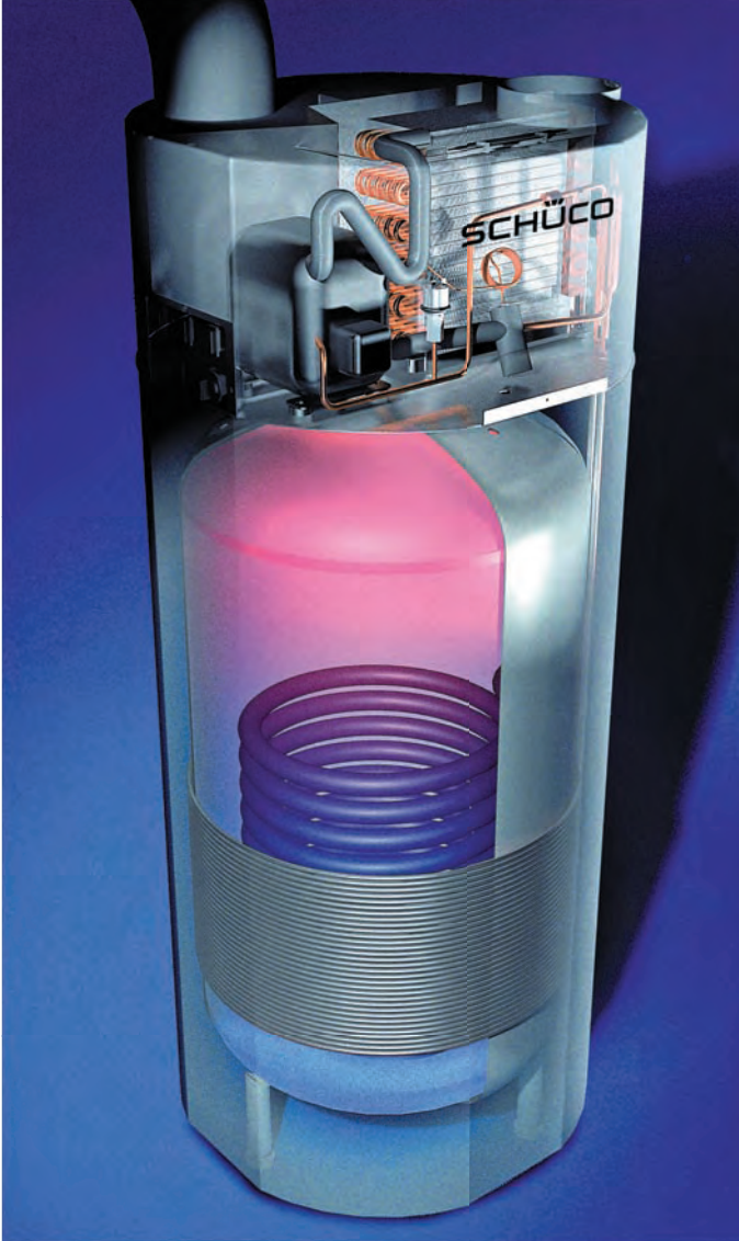
Abb. 5.4: Schnittbild einer solargestützten Wärmepumpe (Grafik: Schüco)
