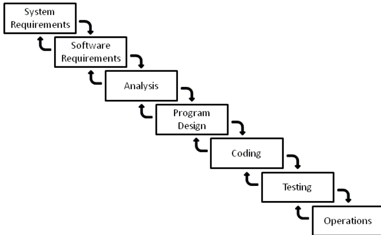
Abbildung 2.1: Erweitertes Wasserfallmodell aus [Roy70]
