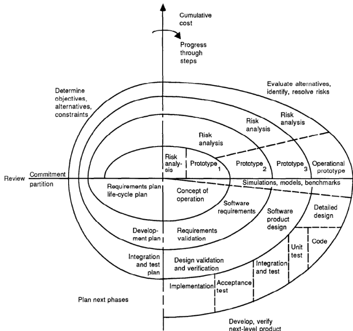
Abbildung 2.3: Spiralmodell aus [Boeh88]
