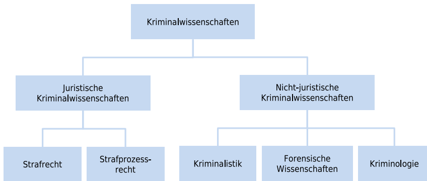
Abb. 1: Kriminalwissenschaften
