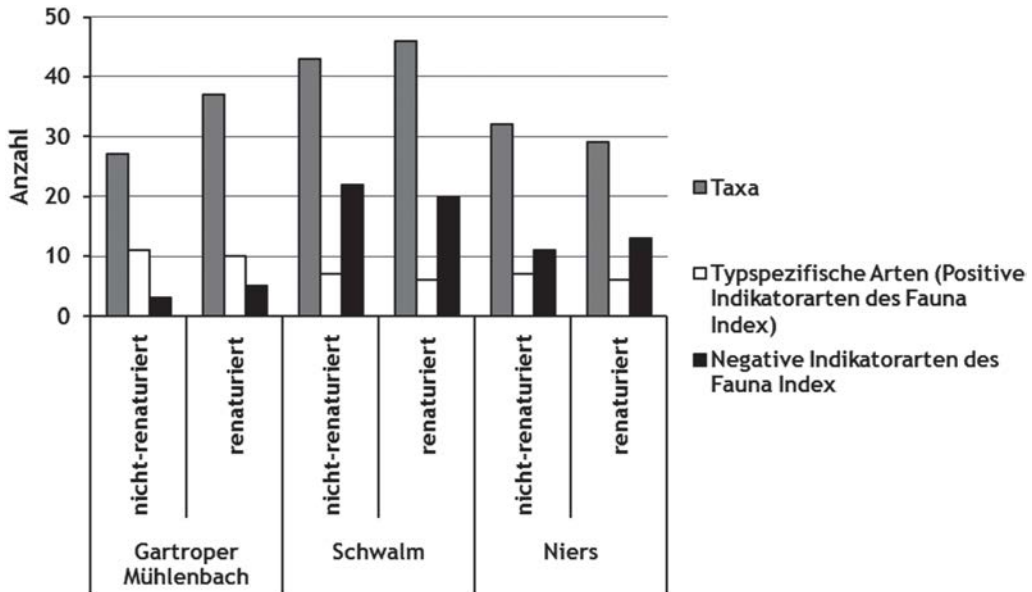
Abb. 1. Taxazahlen, Anzahl typspezifischer Arten und Anzahl negativer Indikatorarten des Makrozoobenthos.
