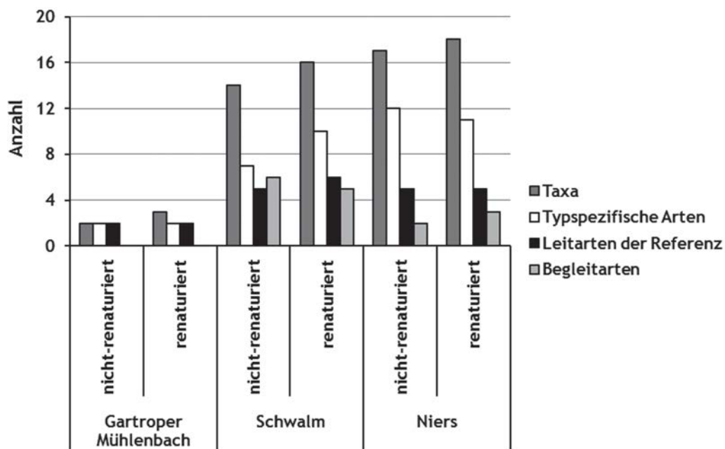
Abb. 3. Taxazahl, Anzahl typspezifischer Arten, Anzahl Leitarten und Anzahl Begleitarten der Fische.
