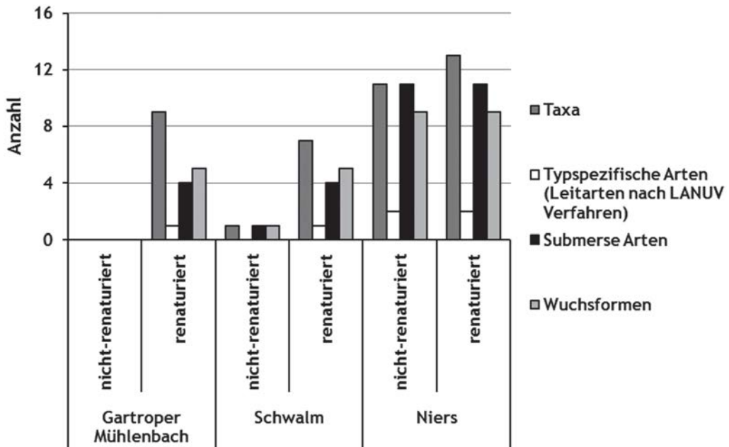
Abb. 5. Taxazahlen, Anzahl typspezifischer Arten (LANUV-Verfahren), Anzahl submerser Arten und Anzahl Wuchsformen der Makrophyten.
