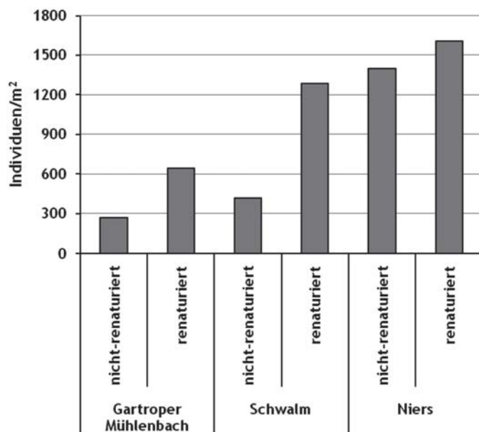
Abb. 2. Abundanzen des Makrozoobenthos (Ind./m²).
