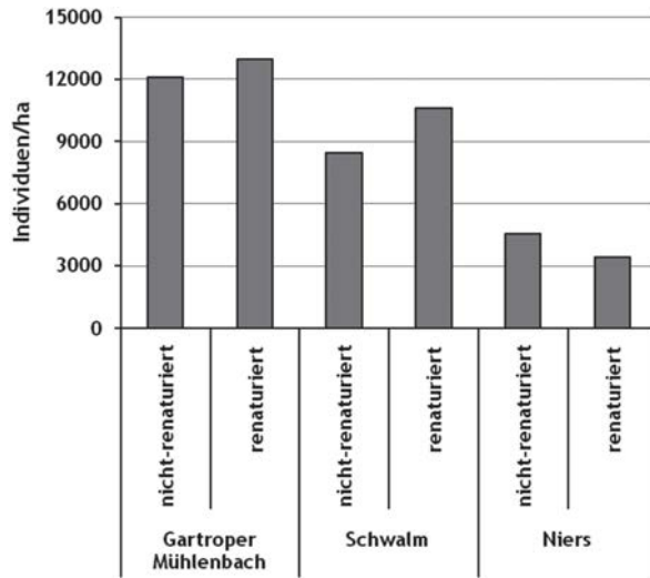
Abb. 4. Abundanzen der Fische (Ind./ha).
